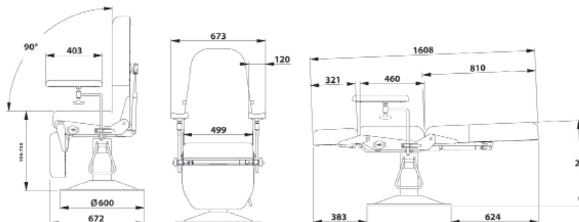
HAUTEUR VARIABLE HYDRAULIQUE / HYDRAULIC HEIGHT ADJUSTMENT
