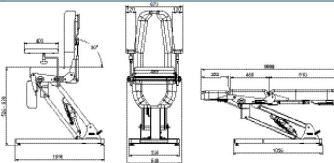
HAUTEUR VARIABLE HYDRAULIQUE / HYDRAULIC HEIGHT ADJUSTMENT
