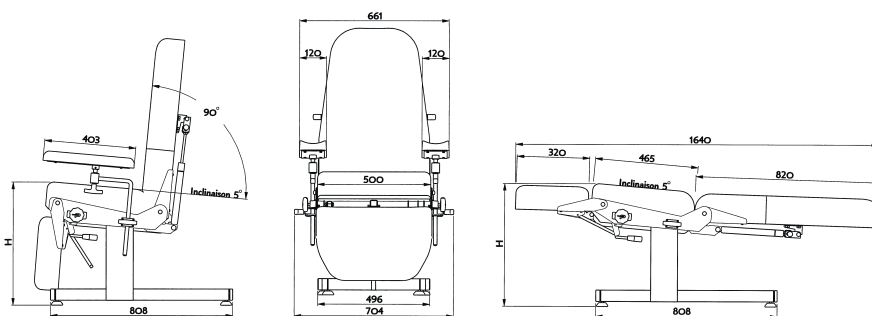
HAUTEUR VARIABLE ÉLECTRIQUE / ELECTRIC HEIGHT ADJUSTMENT
